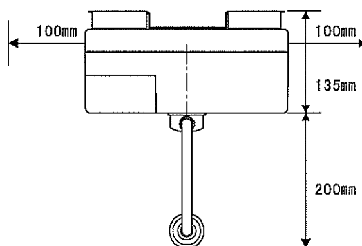
● 本体平面図
